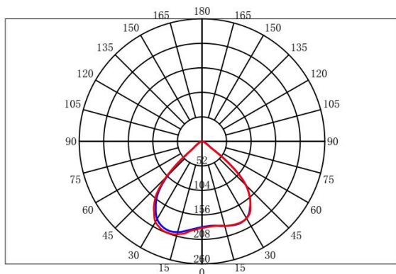
配光曲线
